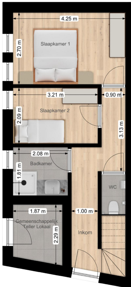
Blok 1 - Gelijkvloers
